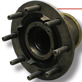
8 Stud 275PCD 90578
