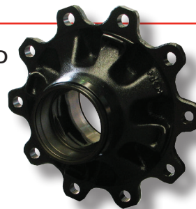
BPW ECO + ECO Plus 10 Stud 335 PCD 0327243120
